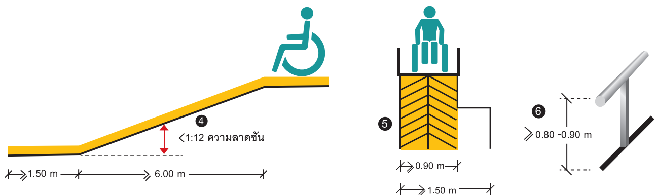
รูปที่ 14 : สัดส่วนทางลาดสำหรับคนพิการใช้รถเข็นนั่ง
