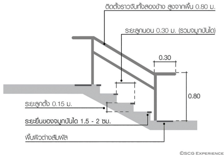
รูปที่ 18 : แสดงสัดส่วนขนาดบันได
